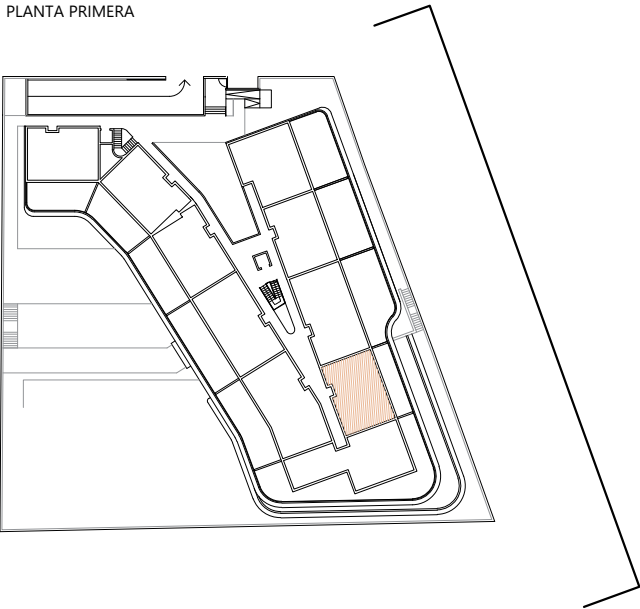
PLANTA PRIMERA
