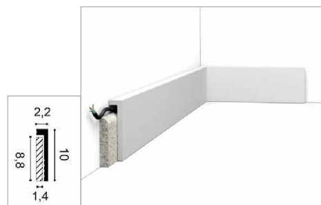
CUBRERODAPIE ZÓCALO DE ORAC EN PAREDES EXISTENTES MODELO SX171-RAL9003 SQUARE ALTURA 10 CM
